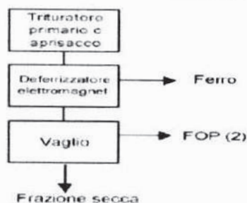
Schema b) (impianto di separazione secco umido)
