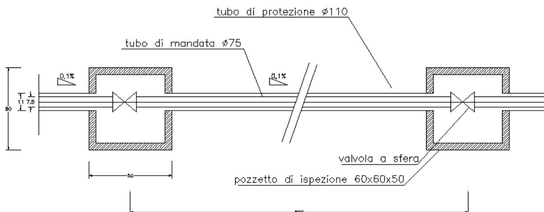
Pozzetti di controllo della tubazione interrata
